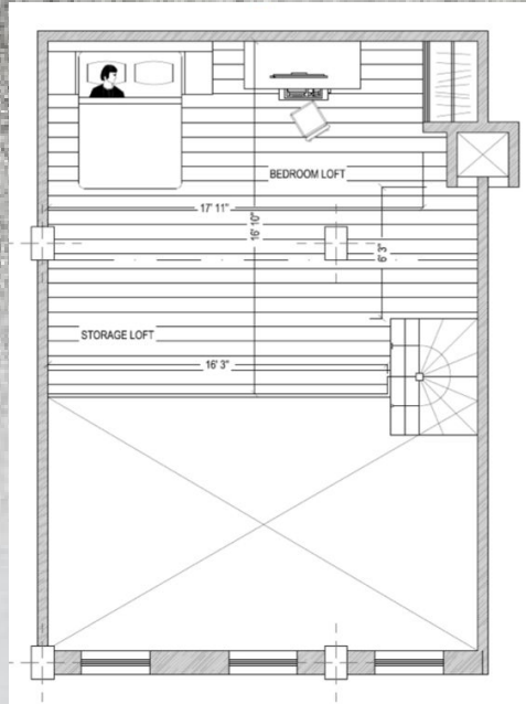
BEDROOM LOFT
